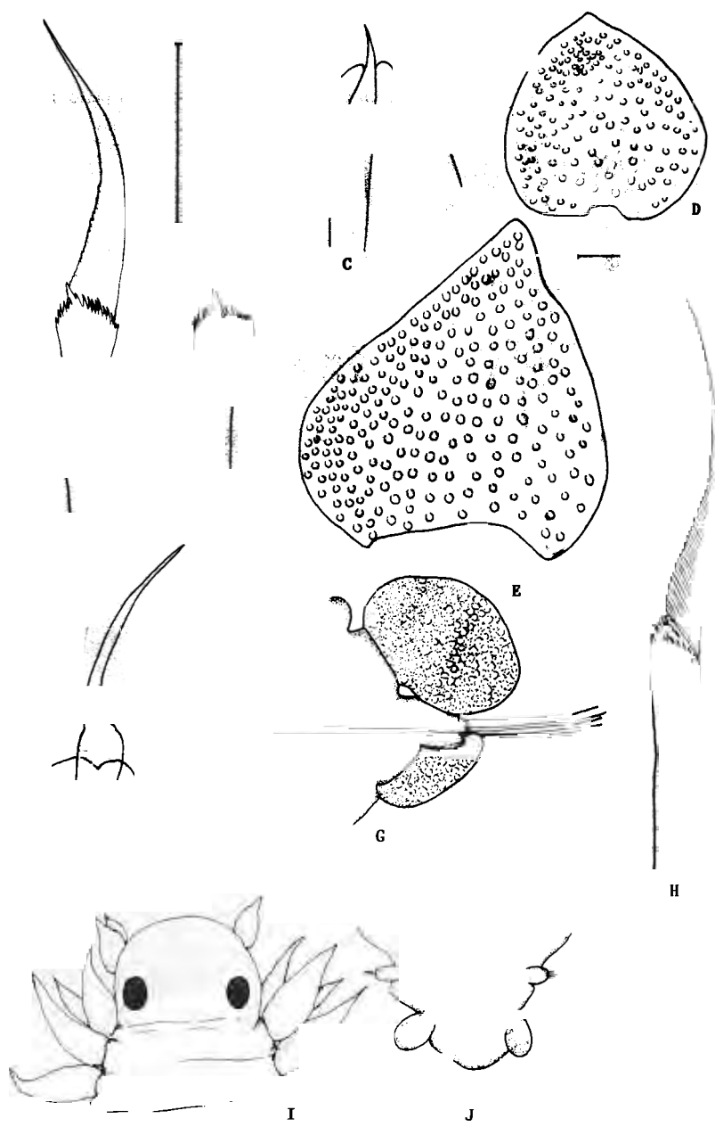
Fig. 2. Nereiphylla rubiginosa : A, seda compuesta espiniforme; B, mango de la seda; C, acícula; D, cirro dorsal anterior; E, cirro dorsal medio. Nereiphylla nana : F, acícula; G, parápodo; H, seda compuesta espiniforme; I, prostomio y segmentos tentaculares (visión dorsal); J, pigidio. Escala: A,B,C,F,H, 20 \mu m; D,E, 50 \mu m; G,I,J, 100 \mu m.
